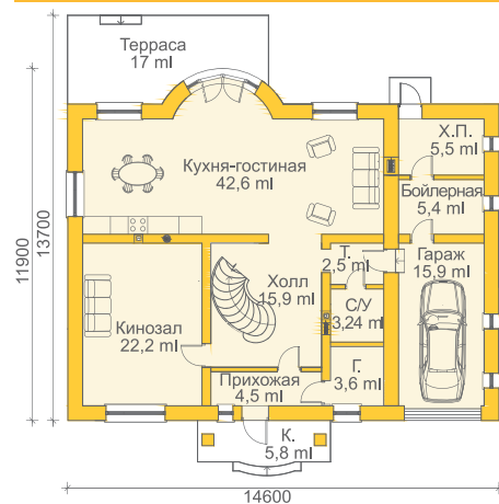
Экспликация | 1 этаж
