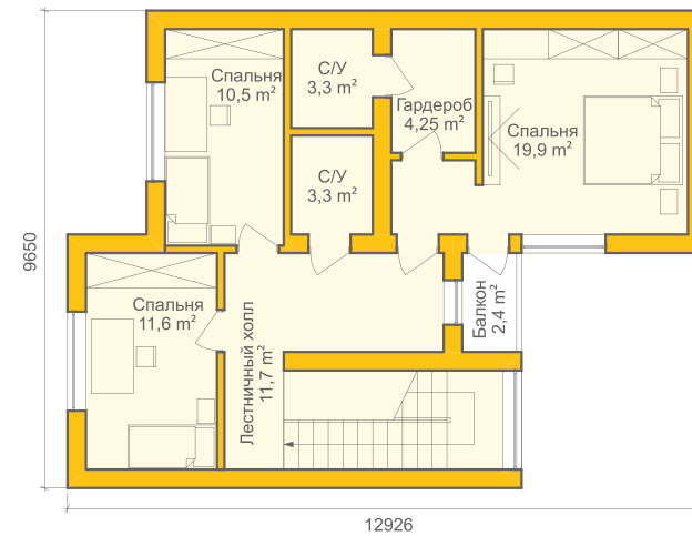
План | 2 этаж
