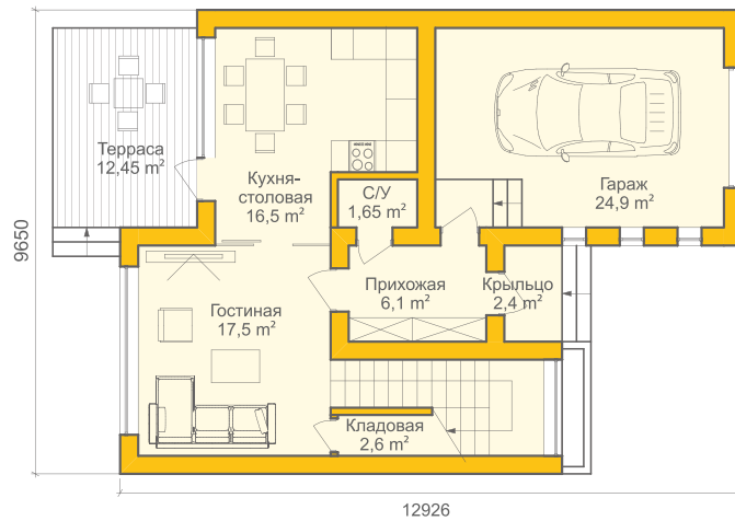
Экспликация | 1 этаж
